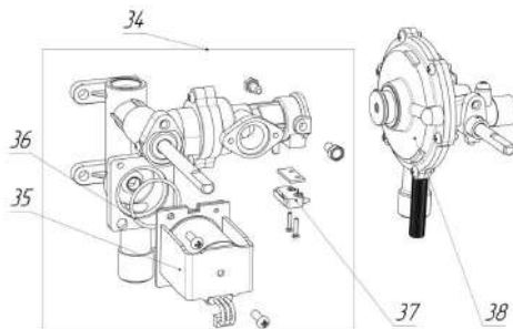
Рисунок 9. Узел водогазовый
