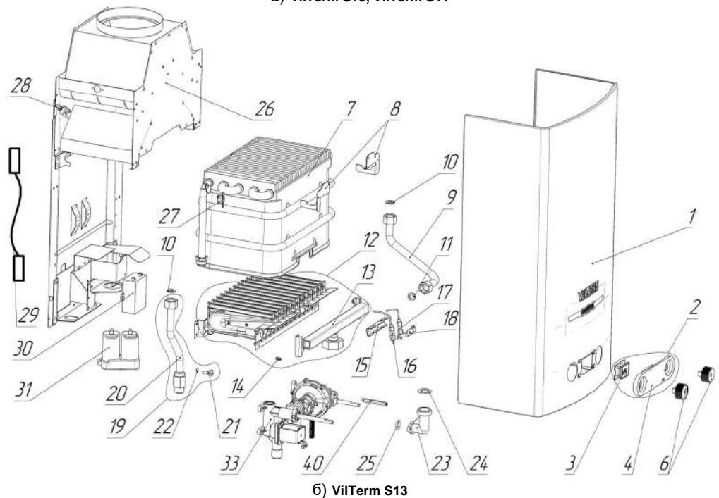
Рисунок 8. Вид аппарата с разнесёнными частями
